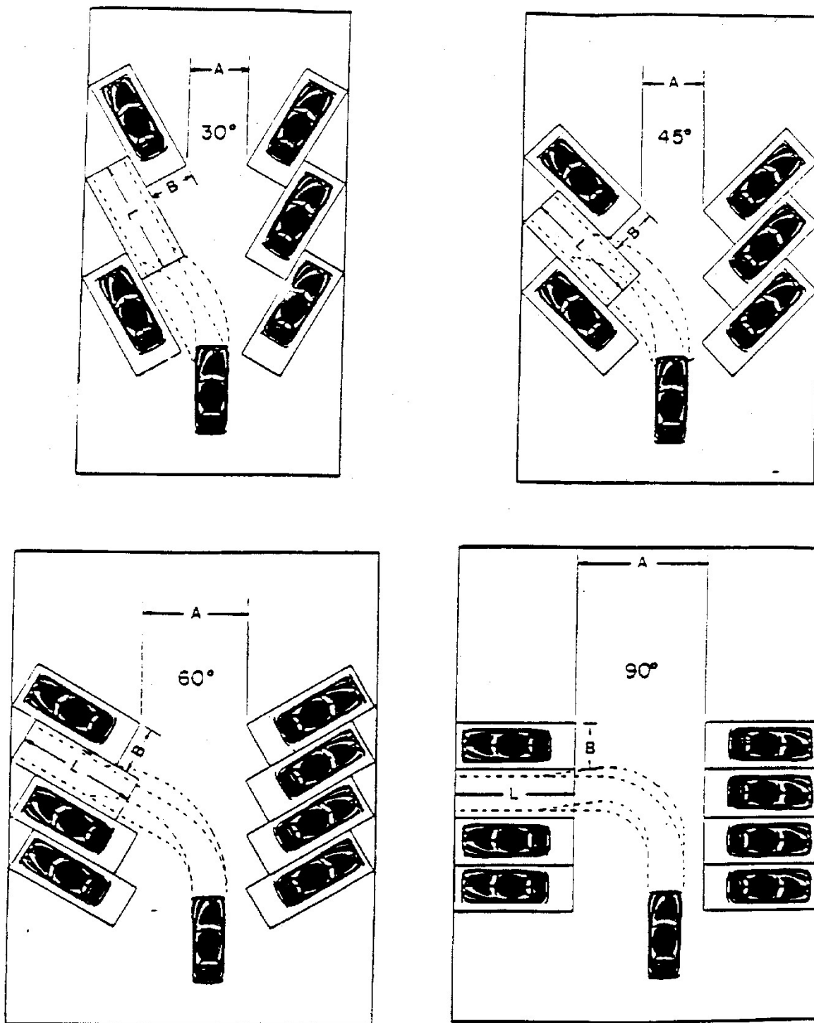
Figure 3 : Dimensions des cases de stationnement et des allées de circulation
